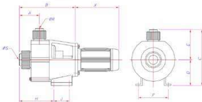
Forma construtiva modelo 160 (Bocais com rosca interna NPT)
