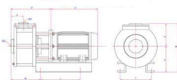
Flange do motor superior a Ø200 (Bocais Norma ANSI ou DIN)
